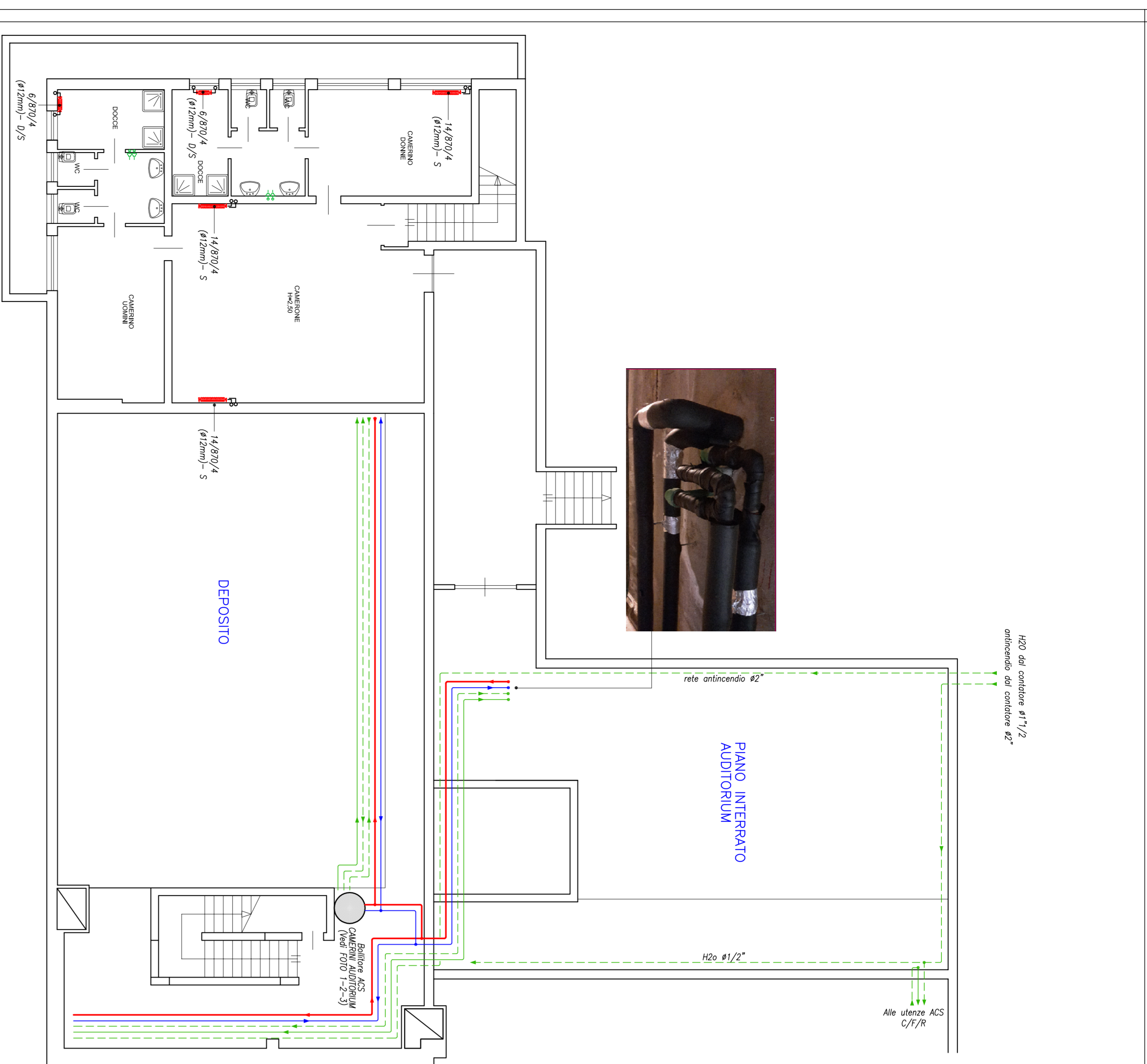
PIANTA PIANO INTERRATO AUTORIUM
